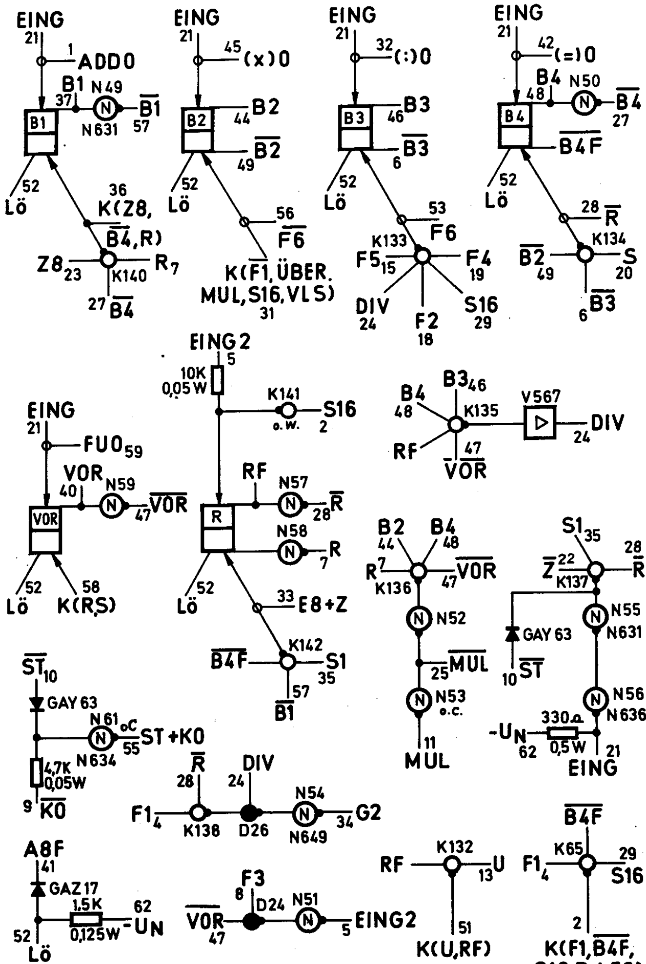
Logischer Plan - Platte 7
